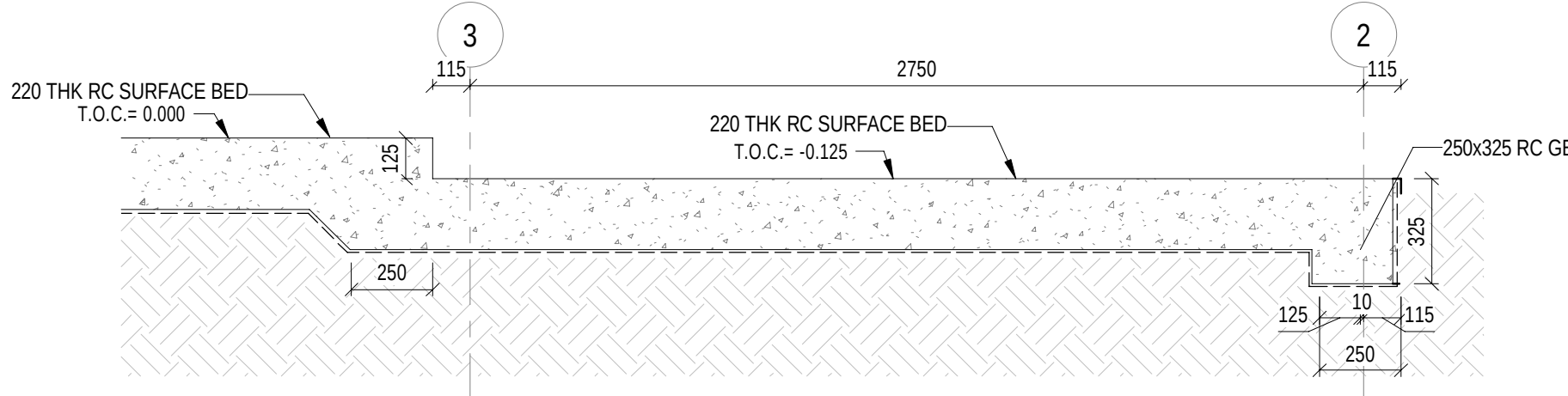
SECTION SC4 - PATIO STEP & EDGE 1:20
